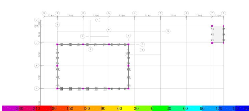
Gambar 9. Pengecekan Tulangan Lantai Atap 2
