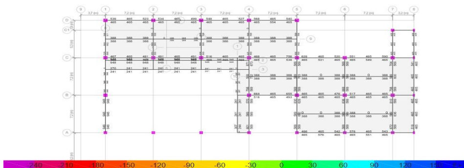
Gambar 8. Pengecekan Tulangan Lantai Atap 1
