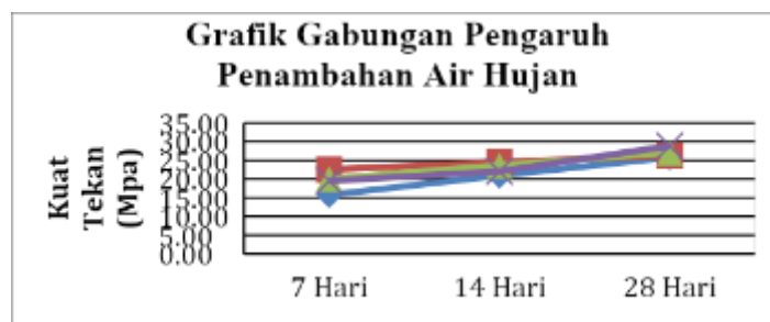
Gambar 9. Grafik Gabungan Variasi Serbuk Cangkang Tiram
