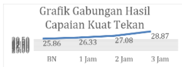
Gambar 10. Grafik Gabungan Hasil Capaian Kuat Tekan
