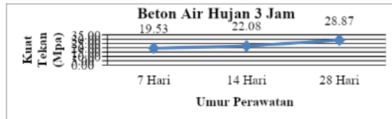
Gambar 9. Grafik pengujian Beton Air Hujan 3 Jam
