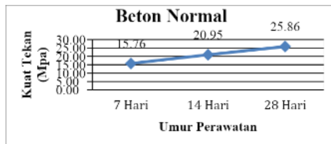
Gambar 6. Grafik pengujian kuat tekan beton normal
