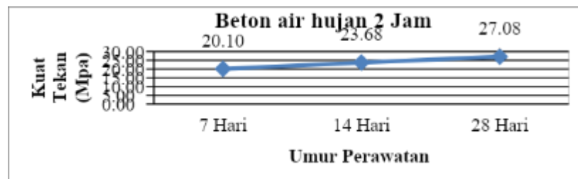
Gambar 8. Grafik pengujian kuat tekan beton air hujan 2 jam
