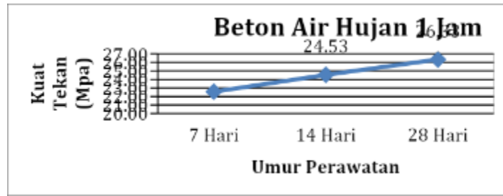
Gambar 7. Grafik pengujian kuat tekan beton air hujan 1 jam
