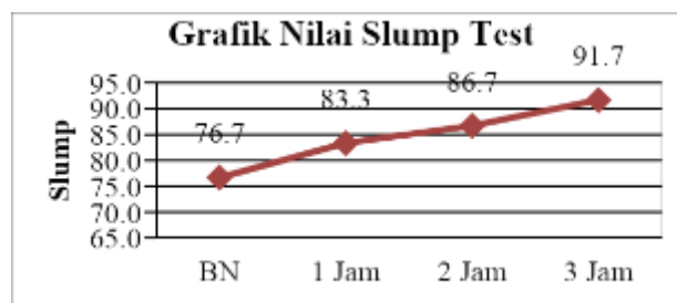
Gambar 5. Perbandingan nilai slump pada setiap variasi
