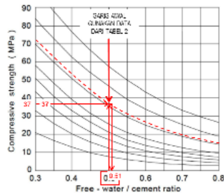
Gambar 3. Grafik perkiraan faktor air semen (Sumber: SNI 03-2834:2000)
