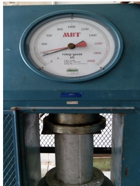
Pengujian kuat tekan beton
