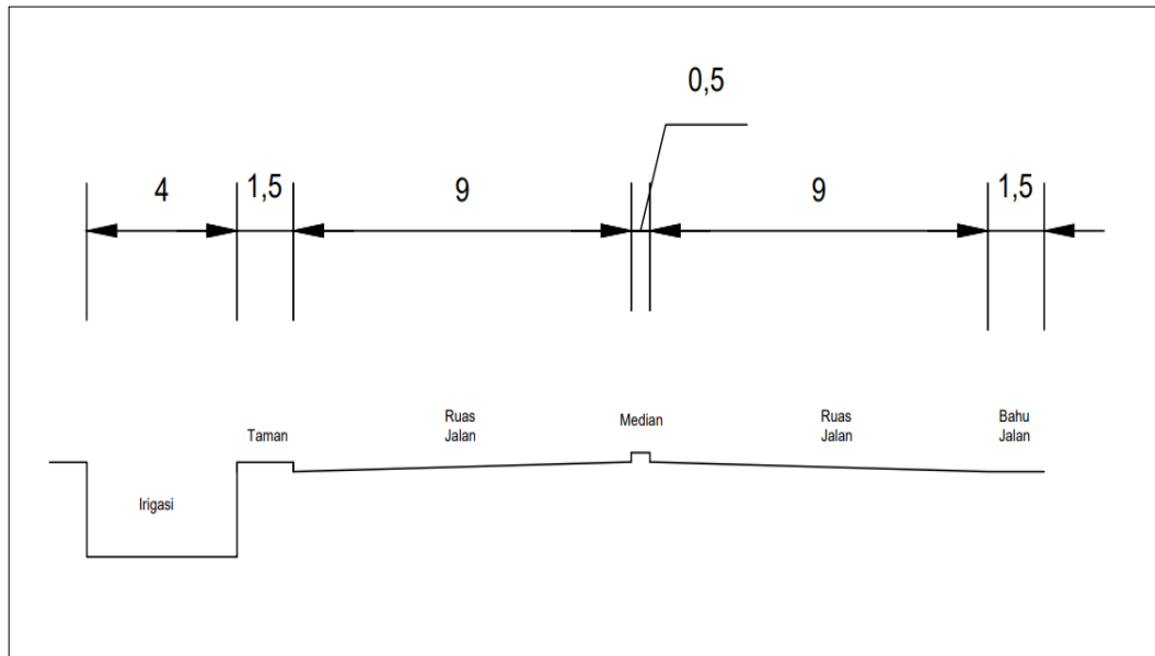
Potongan lokasi penelitian Jl. Bintang
