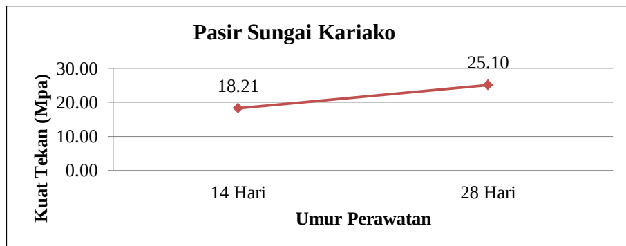
Gambar 3. Grafik Pengujian Kuat Tekan Beton Normal
