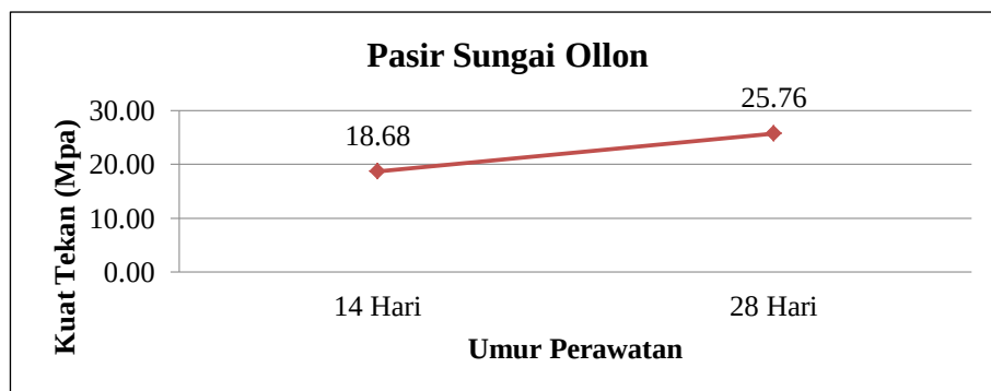
Gambar 4. Grafik Pengujian Kuat Tekan Beton Pasir Sungai Ollon
