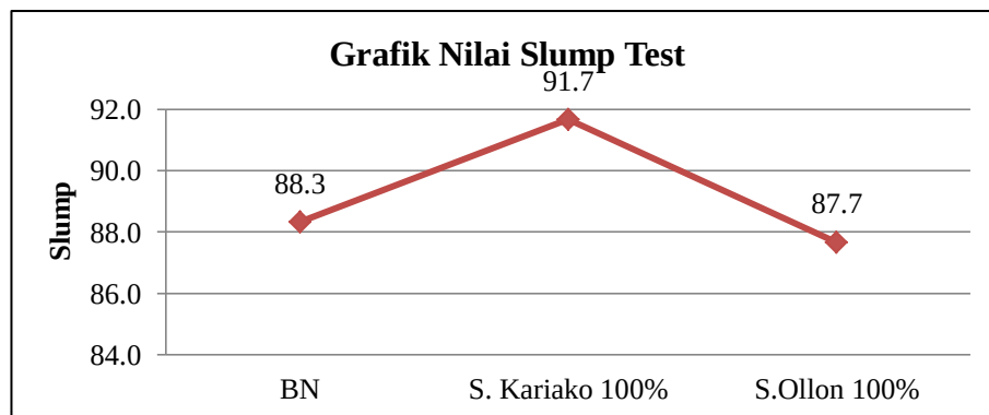
Gambar 1. Perbandingan Nilai Slump Pada Setiap Variasi
