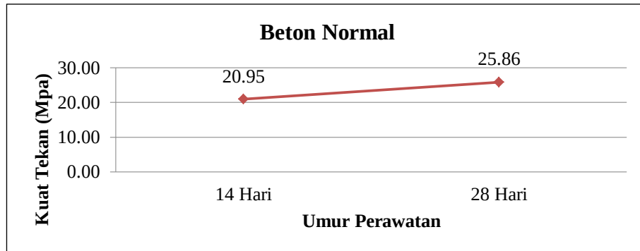
Gambar 2. Grafik Pengujian Kuat Tekan Beton Normal
