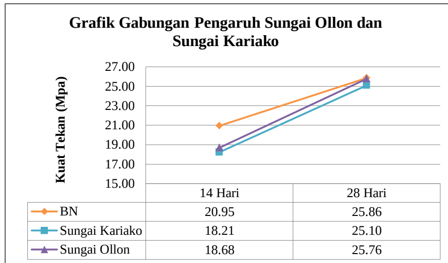
Gambar 5. Grafik Gabungan Pengaruh Pasir Sungai Kariako dan Pasir Sungai Ollon
