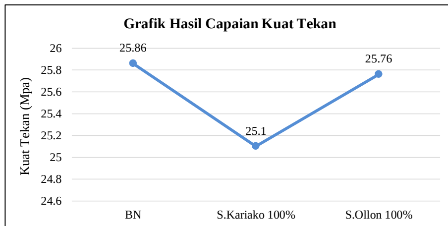
Gambar 6. Grafik Gabungan Hasil Capaian Kuat Tekan
