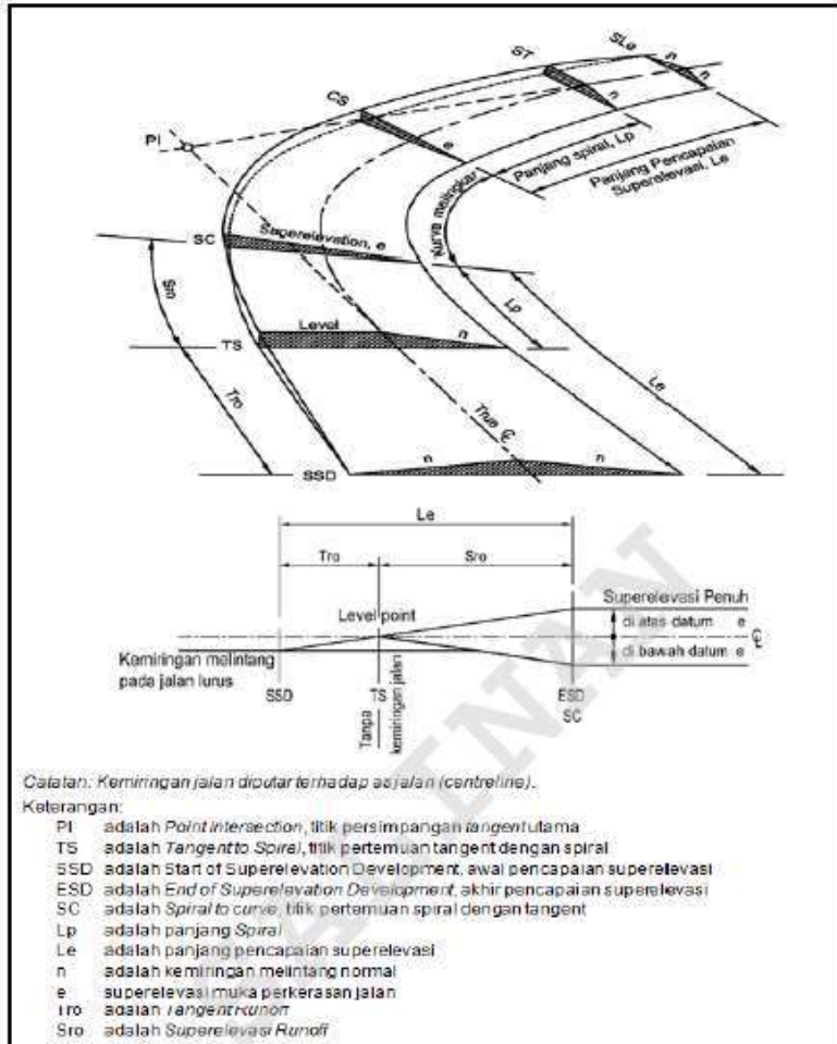
Gambar 9.4. Bentuk tipikal pencapaian superelevasi pada jalan dua lajur (Sumber: Pedoman Desain Geometrik Jalan 2021)
