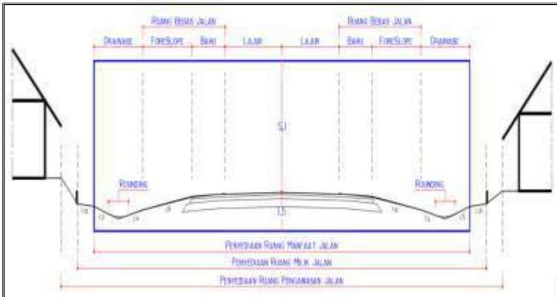
Gambar 2.1. Bagian-bagian jalan
