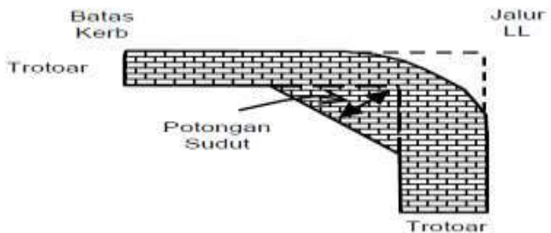
Gambar 10.3. Potongan Sudut
