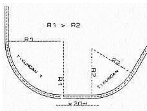
Gambar 5.5. Tikungan Gabungan Searah
