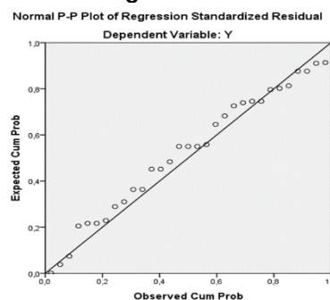
Gambar 1 Uji Normalitas dengan Teknik Probability Plot
