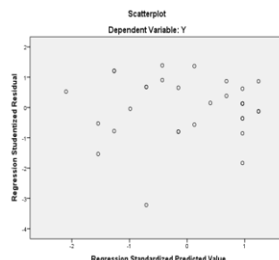
Gambar 2. Uji Heterokedastisitas – Grafik Scatter Plot
