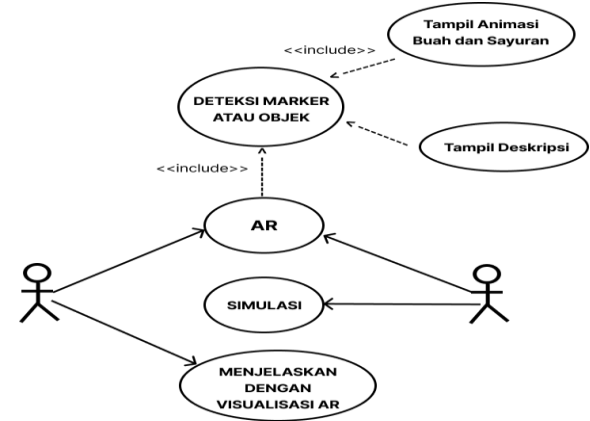
Gambar 2. Desain Sistem yang di usulkan Dan berikutnya Activity Diagram untuk , Scan qr code , Scan gambar dan Latihan :
